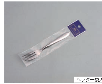
3831 K・K(キャサリン・クライン) 8-24-10 ステン ケーキフォーク ●材質/18-0ステンレス ●商品サイズ/約 142mm 板厚2.0mm ●パッケージサイズ/180×40mm ●カートンサイズ/285×235×180mm ●重量/13kg ●入数/600 (20×30)
