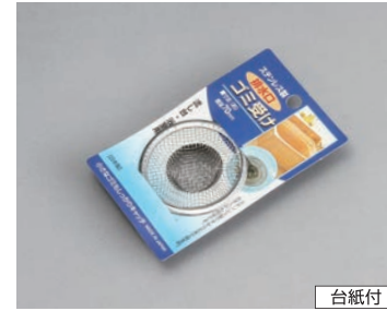
0232 ステンレス排水口ゴミ受け 70mm 8-20-02 ●材質/アミ: 18-8ステンレス鋼 枠: ステンレス鋼 ●商品サイズ/約 φ70×深さ21mm ●パッケージサイズ/143×90×21mm ●カートンサイズ/325×190×165mm ●重量/3kg ●入数/200 (20×10)
